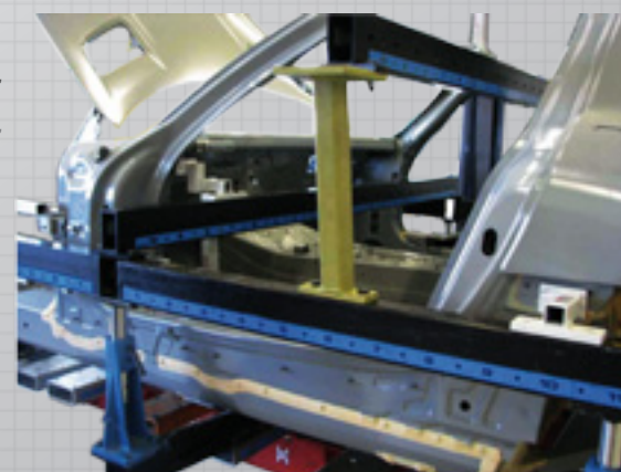
Exemple d'utilisation avec un cabriolet In situation with cabriolet
