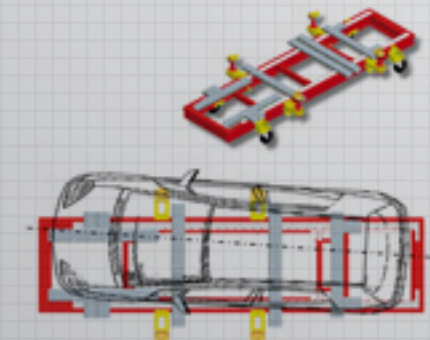
Exemple d'utilisation avec Sevenne uniquement sur les 4 pinces d'ancrage. Measuring with Sevenne only on 4 anchoring clamps
